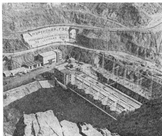
Нурекская ГЭС. 30 сентября введена на полную мощность — 2700 тыс. киловатт.
