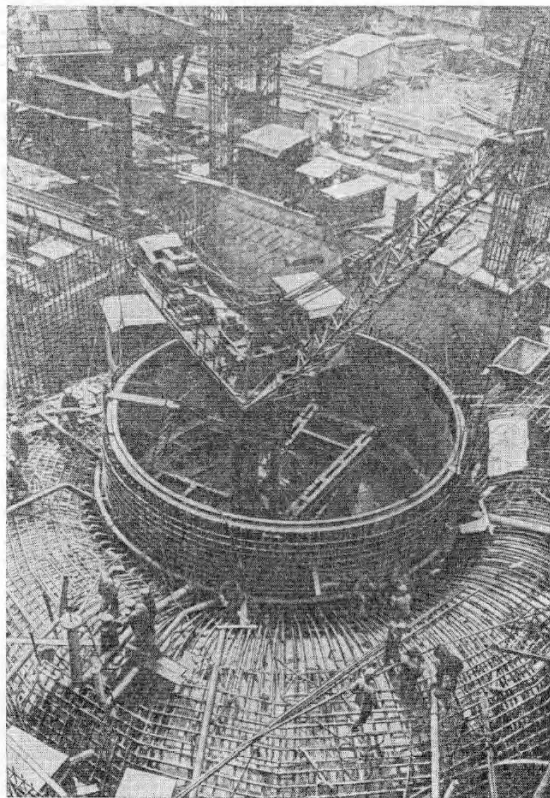
Сооружение спиральной камеры 3-го гидроагрегата Саяно-Шушенской ГЭС.
