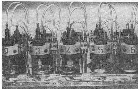
Рис. 3. Малогабаритные манипуляторы.
