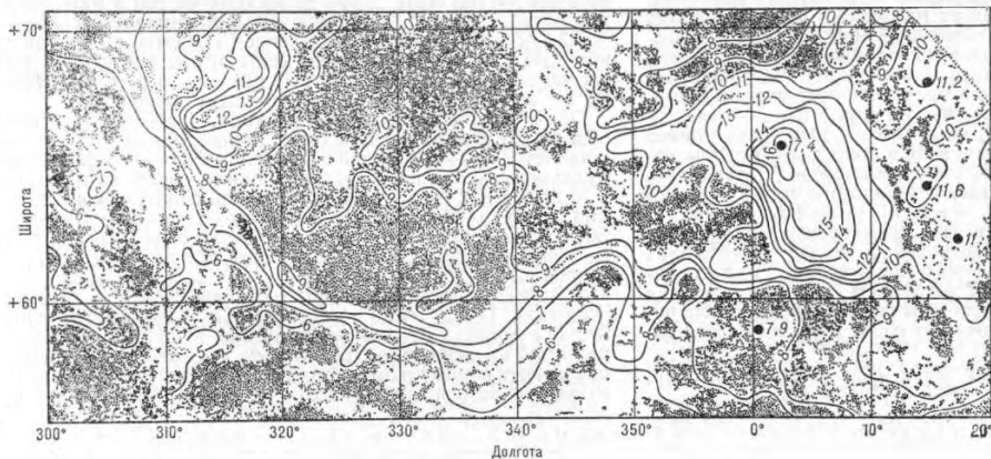
Рис. 8. Топографическая карта части поверхности Венеры по данным наземного радиотелескопа в Аресибо, работавшего в режиме активной локации, и радиокартографа АМС «Пионер-Венера-1». Горизонталы (результат измерений радиокартографа) проведены на карте через 1 км относительно произвольно выбранного радиуса планеты 6045 км. Справа на карте видна светлая область, в которой расположена гора Максвелл (отметка 17,4).
