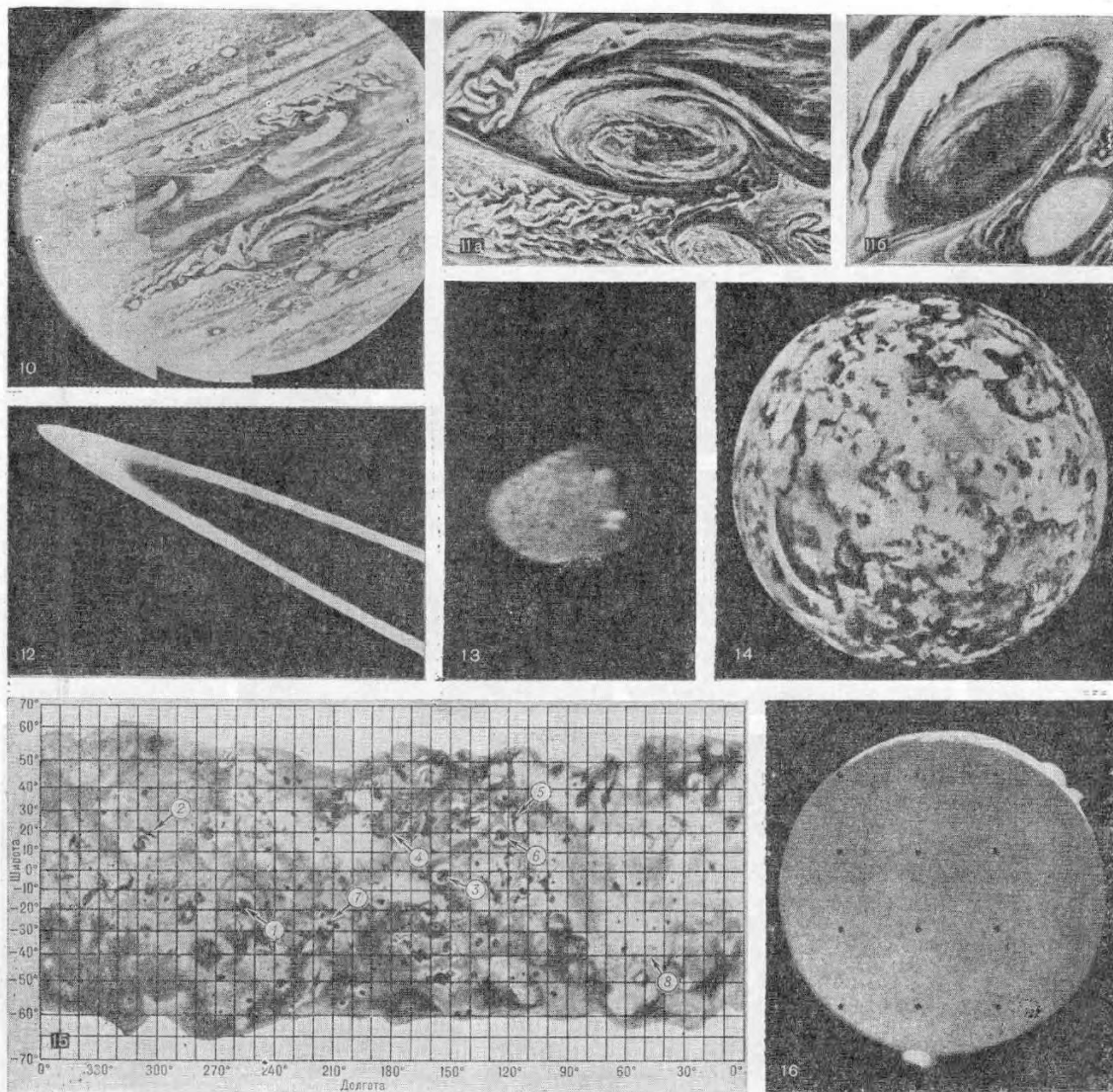
Рис. 10. Мозаичное изображение Юпитера, составленное из снимков, полученных АМС «Вояджер-1» с расстояния 7,8 млн. км (разрешение при съемке атмосферных образований ок. 140 км). Рис. 11. Снимки Красного пятна, полученные АМС «Вояджер-1» (а) и «Вояджер-2» (б). Рис. 12. Кольцо Юпитера. Рис. 13. Амальтея. Рис. 14. Ио. Рис. 15. Карта Ио, составленная по снимкам АМС «Вояджер» (масштаб ~64 км в 1 мм; стрелки с цифрами указывают на места вулканических выбросов). Рис. 16. Вулканические выбросы на Ио (на снимке видны реперные точки).
