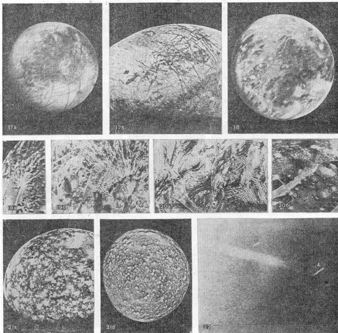
Рис. 17. Европа. Снимки, полученные АМС «Вояджер-1» (а) и «Вояджер-2» (б). Рис. 18. Ганимед. Рис. 19. Ударные кратеры с расходящимися лучами выбросов на Ганимеде, снятые АМС «Вояджер-1» (а) и «Вояджер-2» (б). Рис. 20. Пучки борозд на Ганимеде, снятые АМС «Вояджер-1» (а) и «Вояджер-2» (б). Рис. 21. Каллисто. Снимки, полученные АМС «Вояджер-1» (а) и «Вояджер-2» (б). Рис. 22. Спутник Юпитера 1979-J-1 (А — спутник 1979-J-1; В — звезда; белая полоса — кольцо Юпитера).
