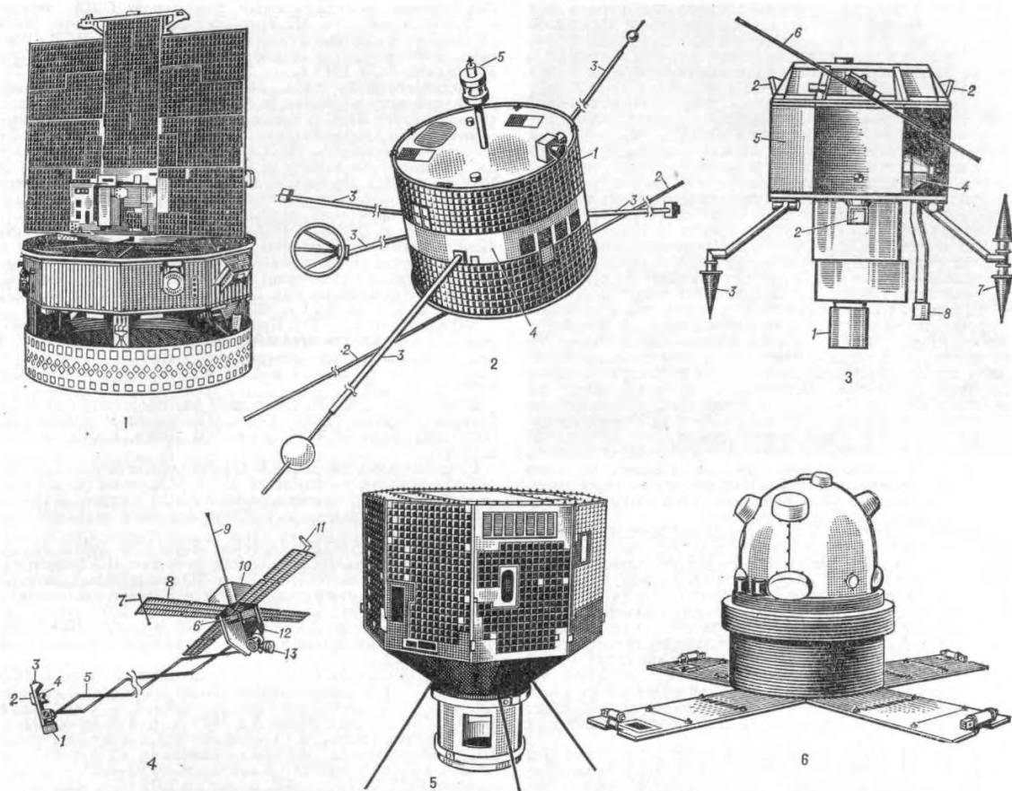
Рис. 1. Спутник «Солуинд». Рис. 2. Спутник SCATHA: 1 — солнечные батареи; 2 — штыри, образующие антенну детектора электрического поля; 3 — штанги с приборами; 4 — корпус; 5 — антенна системы связи. Рис. 3. Спутник «Сейдж»: 1 — фотометр; 2 — солнечные датчики; 3 — антенна для передачи телеметрической информации от научных приборов; 4 — маховики в системе трехосной ориентации; 5 — жалюзи системы терморегулирования; 6 — панель солнечных батарей; 7 — антенна для передачи телеметрической информации о работе бортовых систем; 8 — магнитометр на штанге. Рис. 4. Спутник «Магбат»: 1 — скалярный магнитометр; 2 — векторный магнитометр; 3 — прецизионный солнечный датчик; 4 — уголковые отражатели инфракрасного излучения; 5 — кронштейн для выноса магнитометров; 6 — блок электронного оборудования; 7 — антенна; 8 — панель солнечных батарей; 9 — штанга регулируемой длины для аэродинамической стабилизации; 10 — отсек служебного оборудования; 11 — антенна; 12 — отсек полезной нагрузки; 13 — камеры звездной ориентации. Рис. 5. Спутник «Хакутэ». Рис. 6. Спутник «Аризаль-6».
