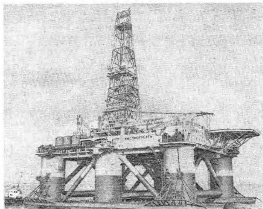
Полупогруженная установка «Каспинефть» пополнила в 1979 г. флотилию плавучих буровых, ведущих поиски нефти в Каспийском море. Она способна вести бурение на участках глубины 200 м (втрое больше, чем доступно обычным буровым).
