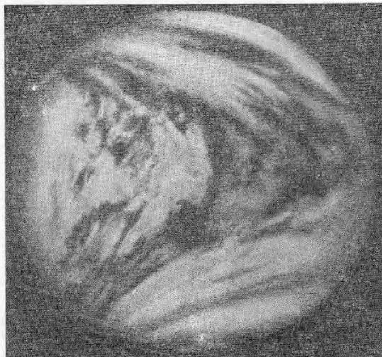
Рис. 7. Изображение облачного покрова полного диска Венеры, полученное АМС «Пионер-Венера-1».
