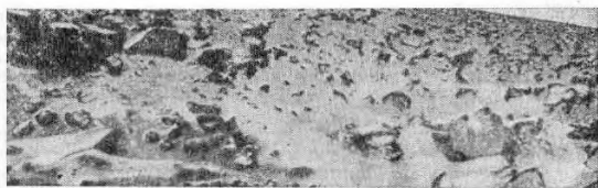
Рис. 9. Снимок поверхности Марса в районе посадки, переданный посадочным блоком АМС «Викинг-2» в начале августа 1979 г.
