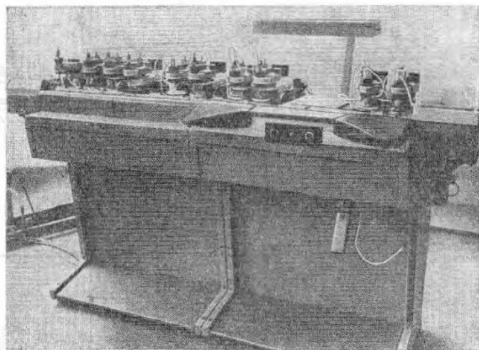
Рис. 2. Сборочный агрегат из двух модулей.
